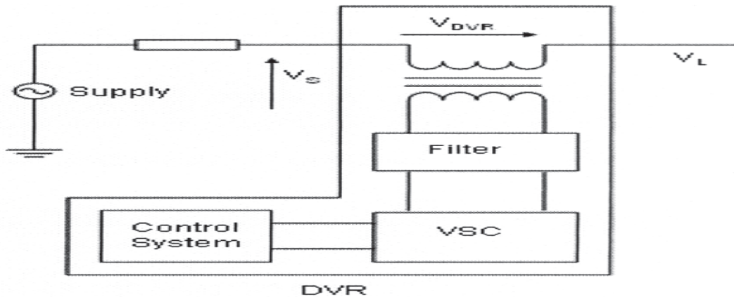
Figure4: Actual schemes of a DVR
